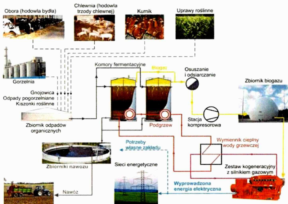
Rysunek 32. Wykorzystanie biogazu z odpadów organicznych [32].
