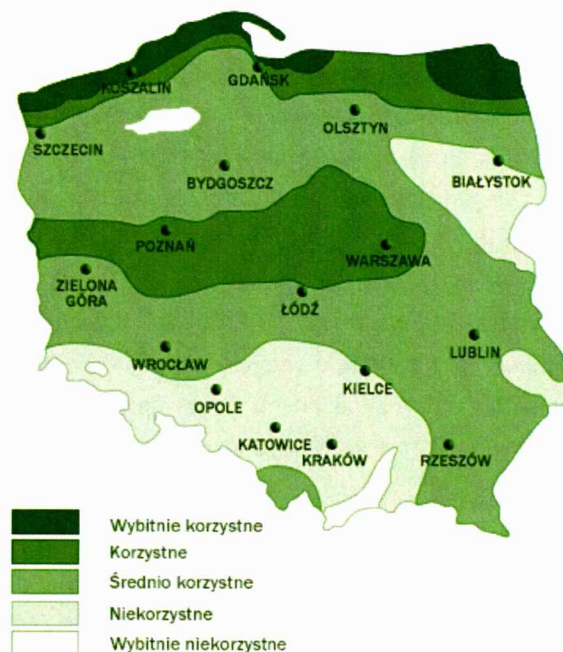
Rysunek 34. Strefy energetyczne warunków wiatrowych [36].
