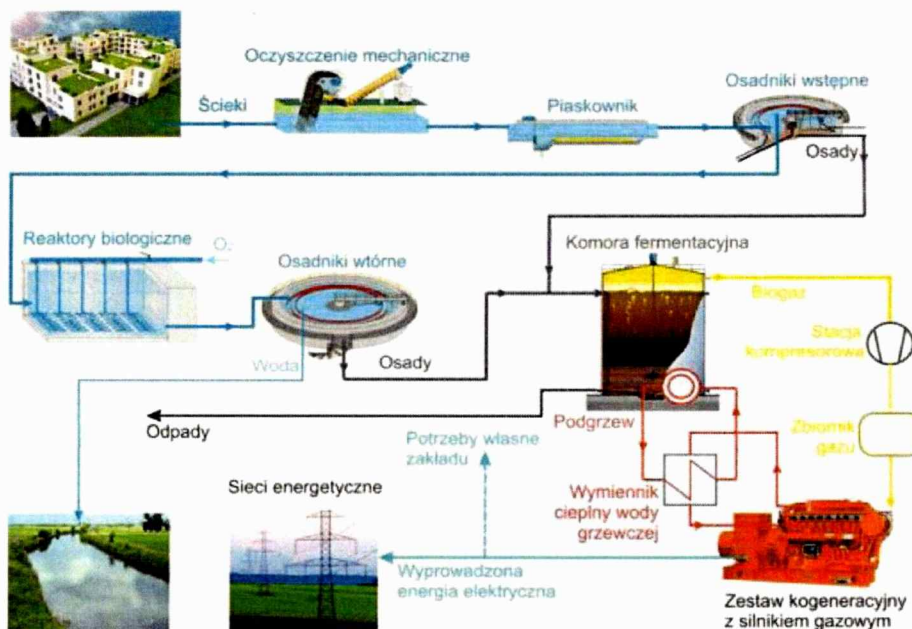
Rysunek 33. Produkcja energii w biogazowni zlokalizowanej przy oczyszczalni ścieków.
