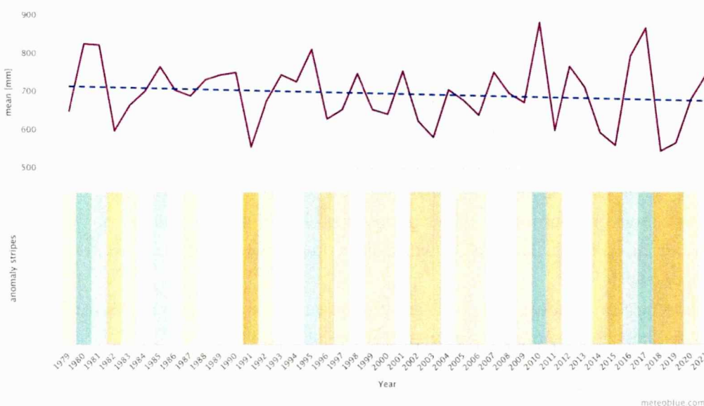
Rysunek 30. Roczna zmiana opadów w Suwałkach [28].
