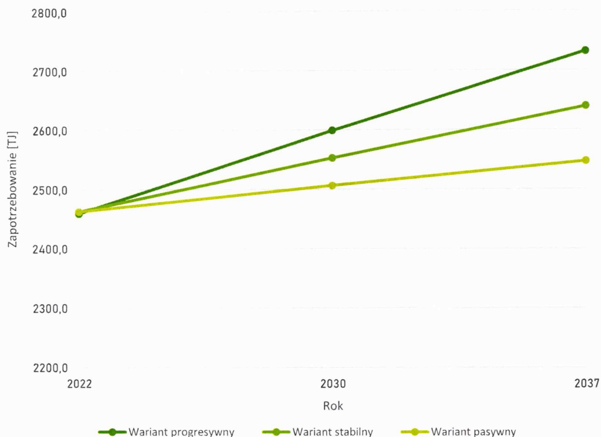
Rysunek 38. Prognozowana zmiana zużycia ciepła do roku 2037.
