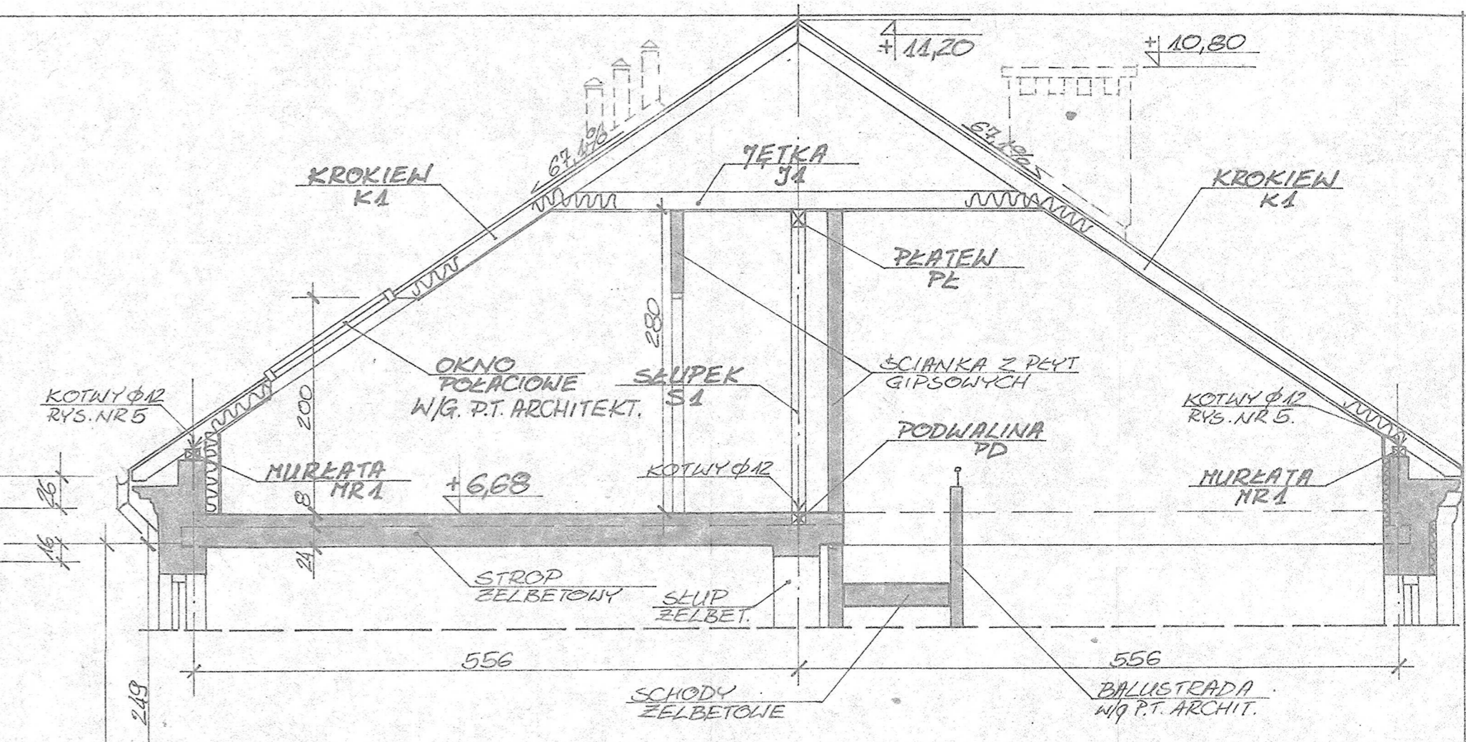
PRZEKRÓJ A-A
