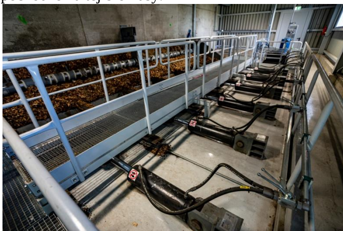
Instalacja podawania biomasy, fot. archiwum PEC w Suwałkach Sp. z o.o
