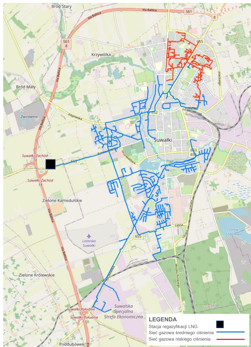
Rysunek 4.2.1 Mapa sieci gazowej w Suwałkach do 30.11.2019 r.
