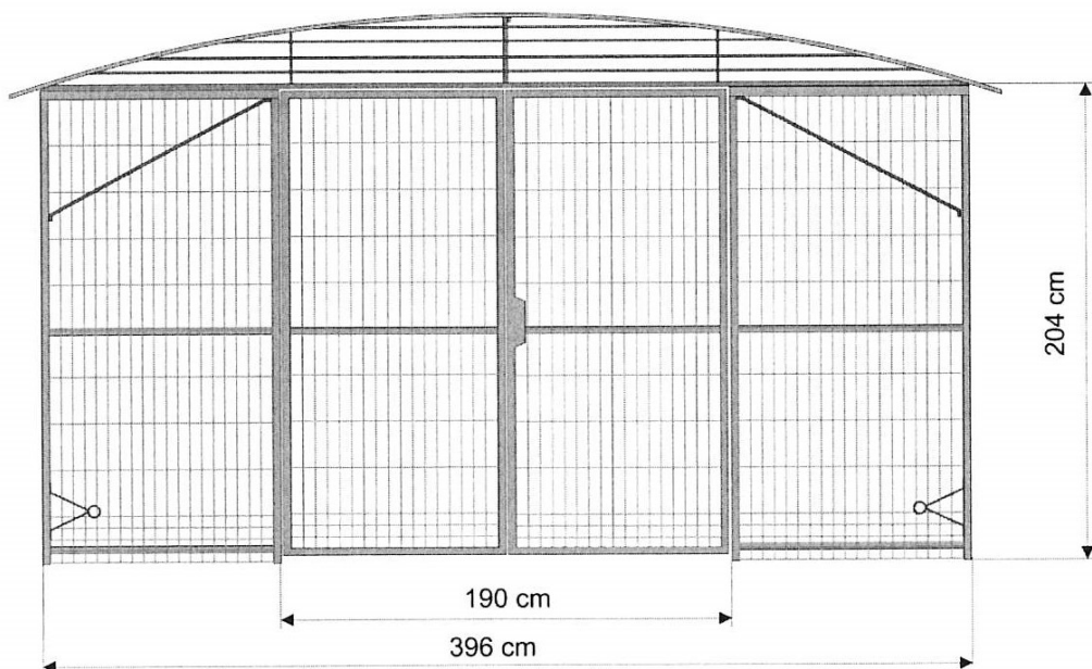
Widok ściany czołowej z furtką dwuskrzydłową.
