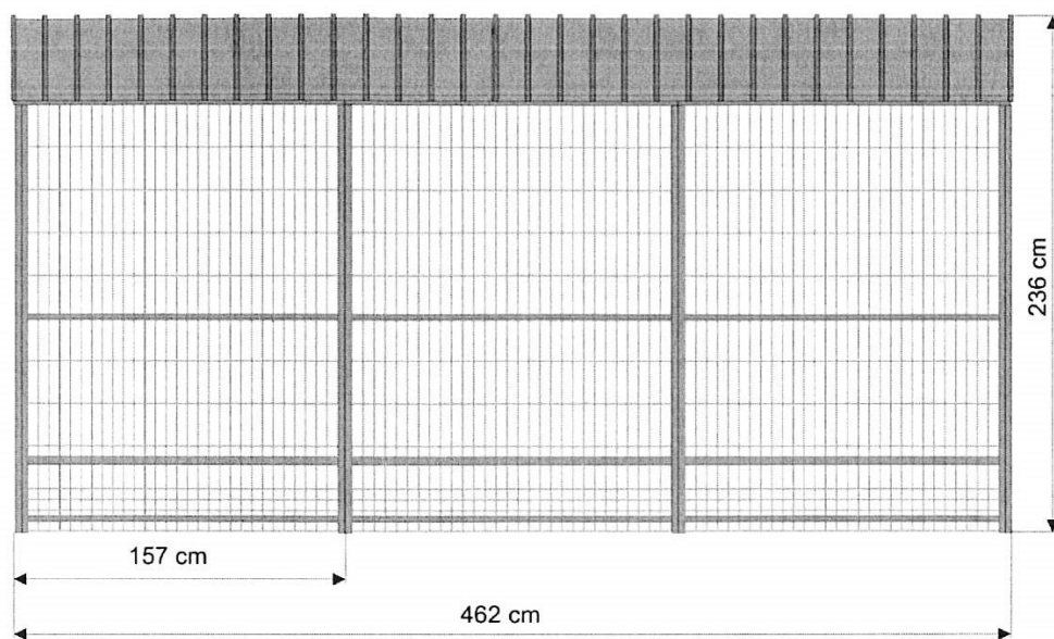
Widok z boku zabudowy na 6 pojemników.
