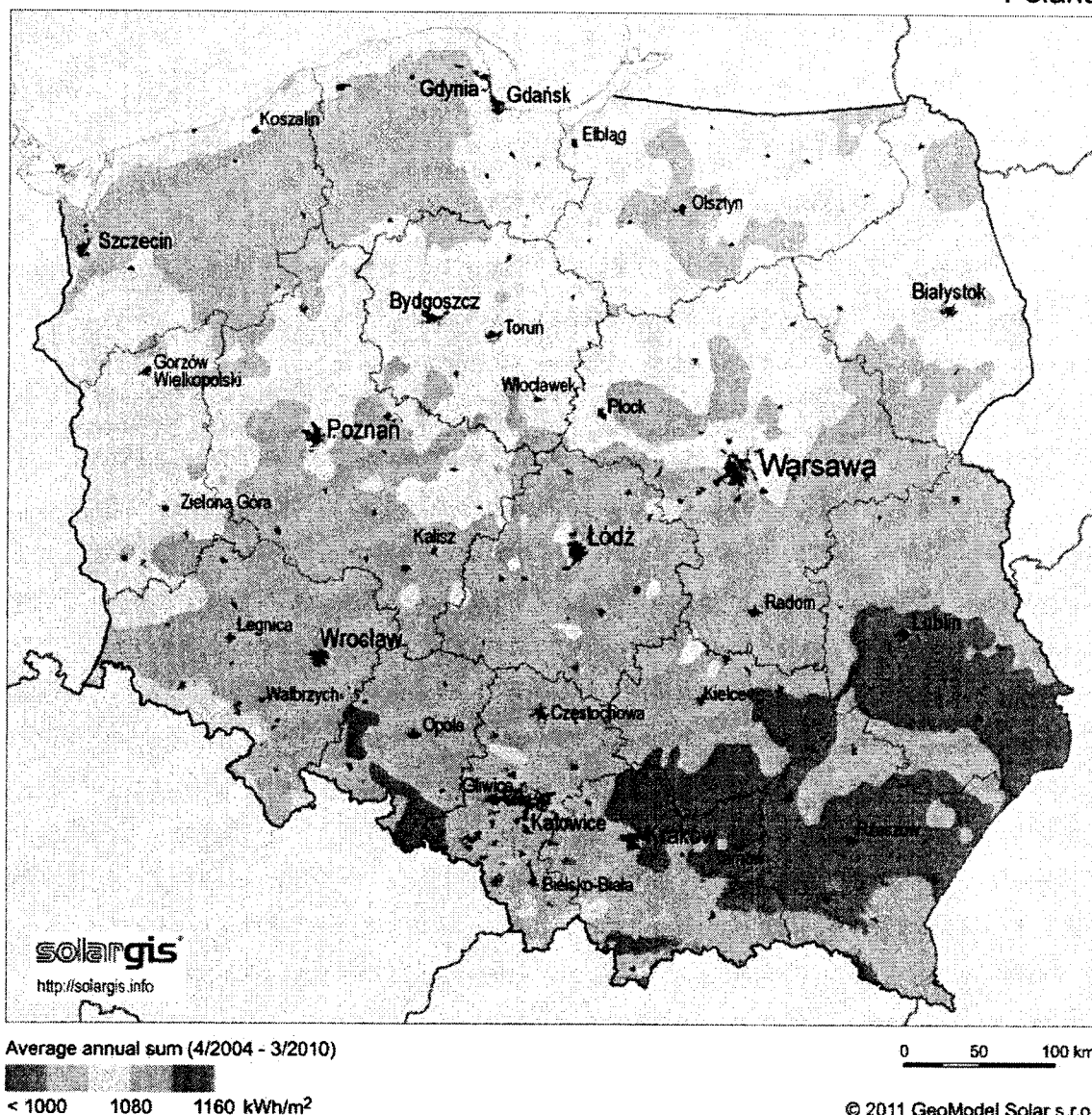
Mapa 4. Nasłonecznienie w Polsce
