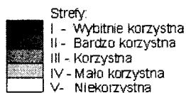
Mapa 5 Strefy energetyczne wiatru w Polsce Źródło: Ośrodek Meteorologii i Gospodarki Wodnej
