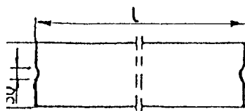
Rys. 1. Wymiarowanie krawężników
