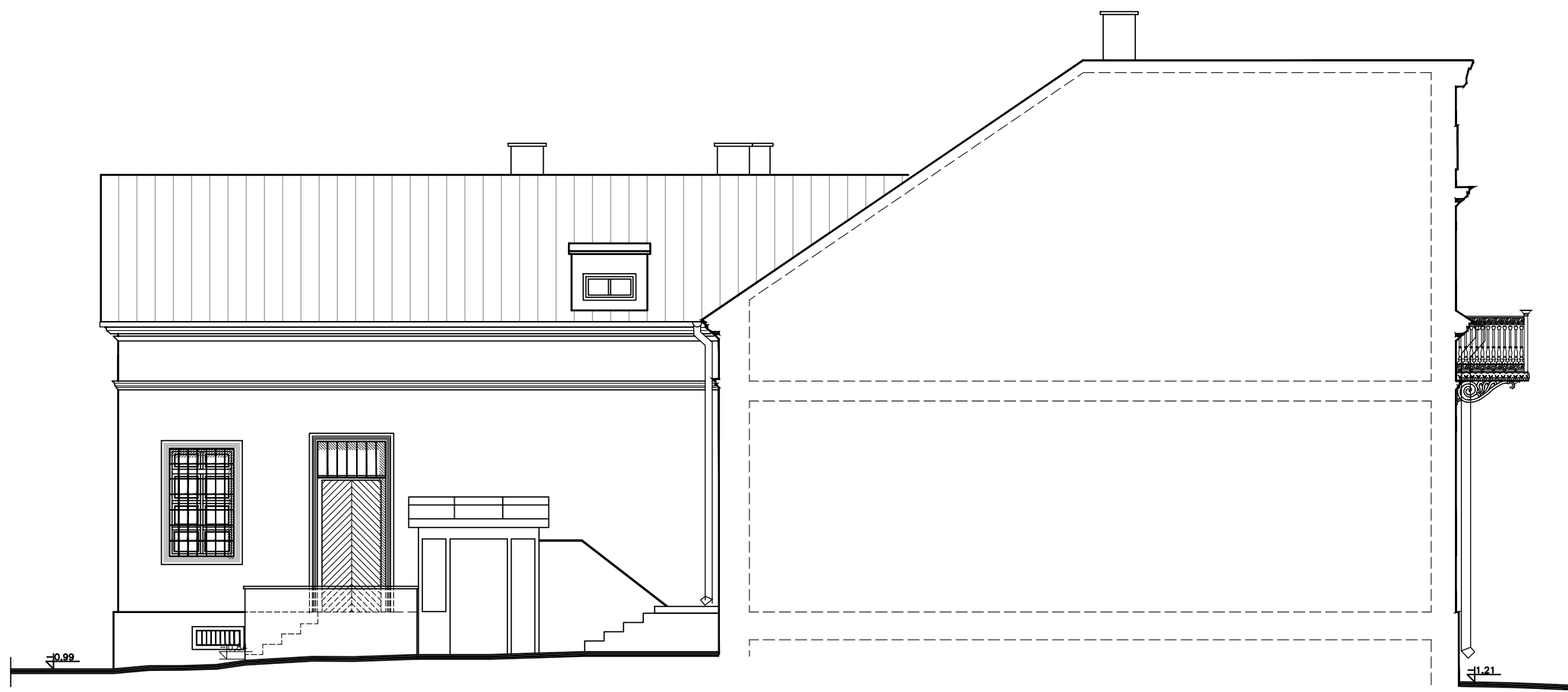
ELEWACJA PÓŁNOCNA OD DZIEDZIŃCA skala 1:100
