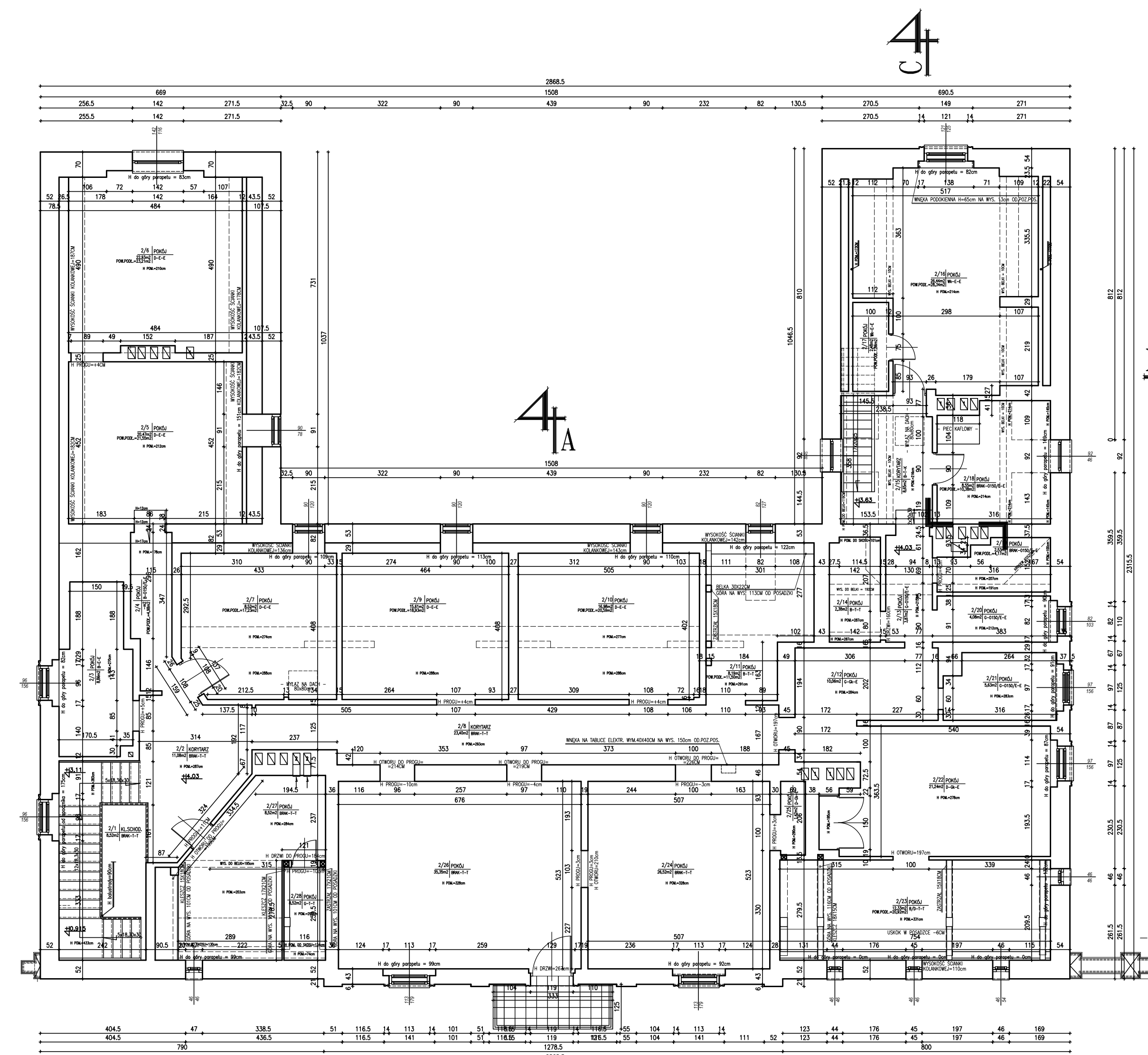
RZUT PODDASZA skala 1:100
