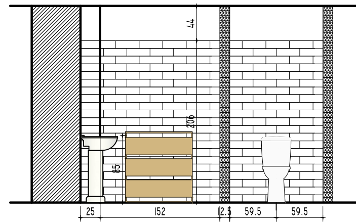
WIDOK B:B
