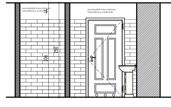
WIDOK C:C
