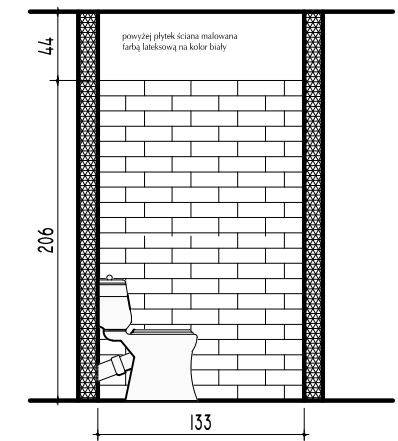
WIDOK D:D
