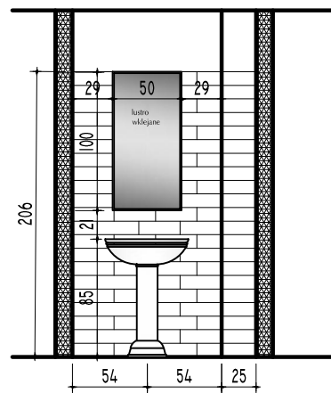
WIDOK A:A
