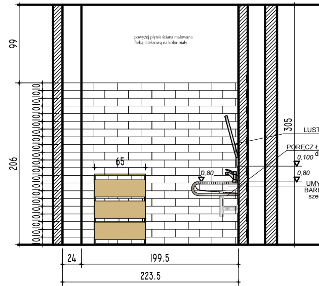
WIDOK A:A
