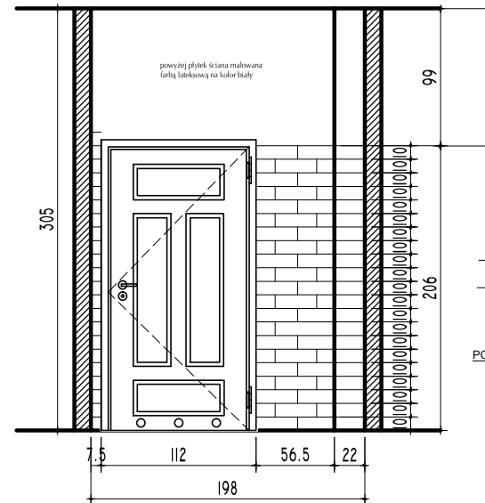
WIDOK B:B
