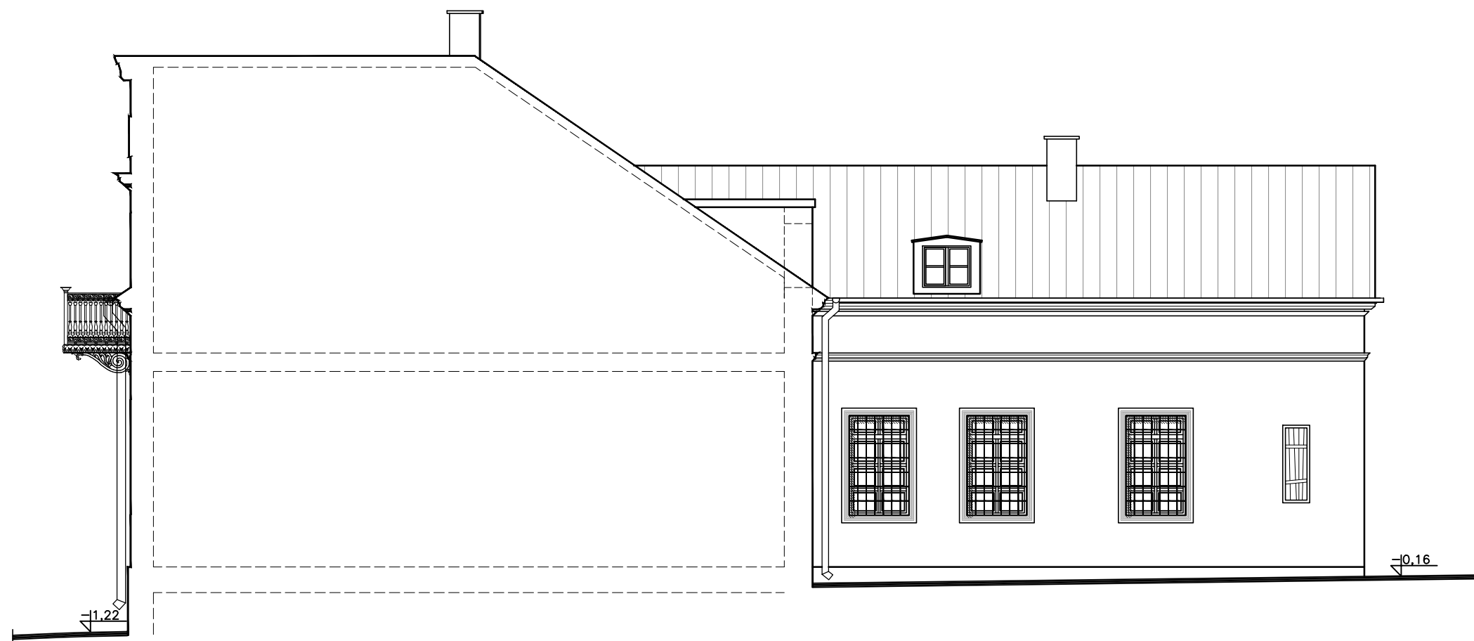
ELEWACJA POŁUDNIOWA OD DZIEDZIŃCA ————— skala 1:100
