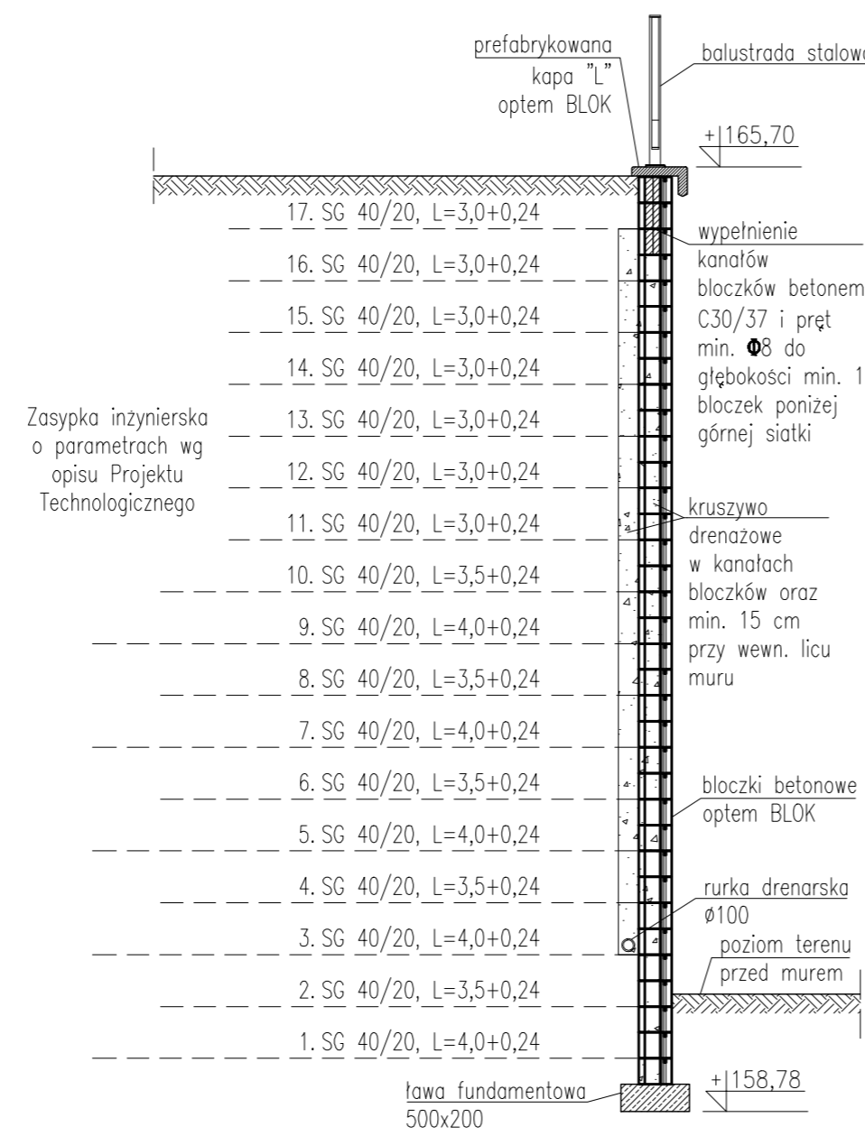
Przekrój B-B skala 1:50
