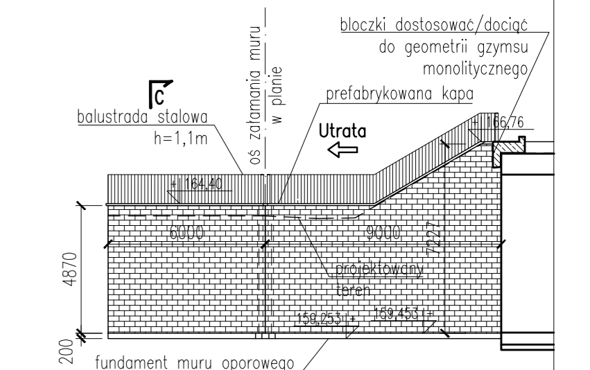
Mur oporowy M02 w rozwinięciu skala 1:200
