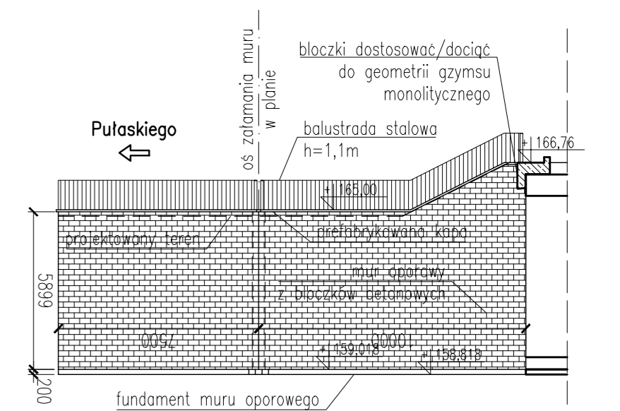
Mur oporowy M03 w rozwinięciu skala 1:200
