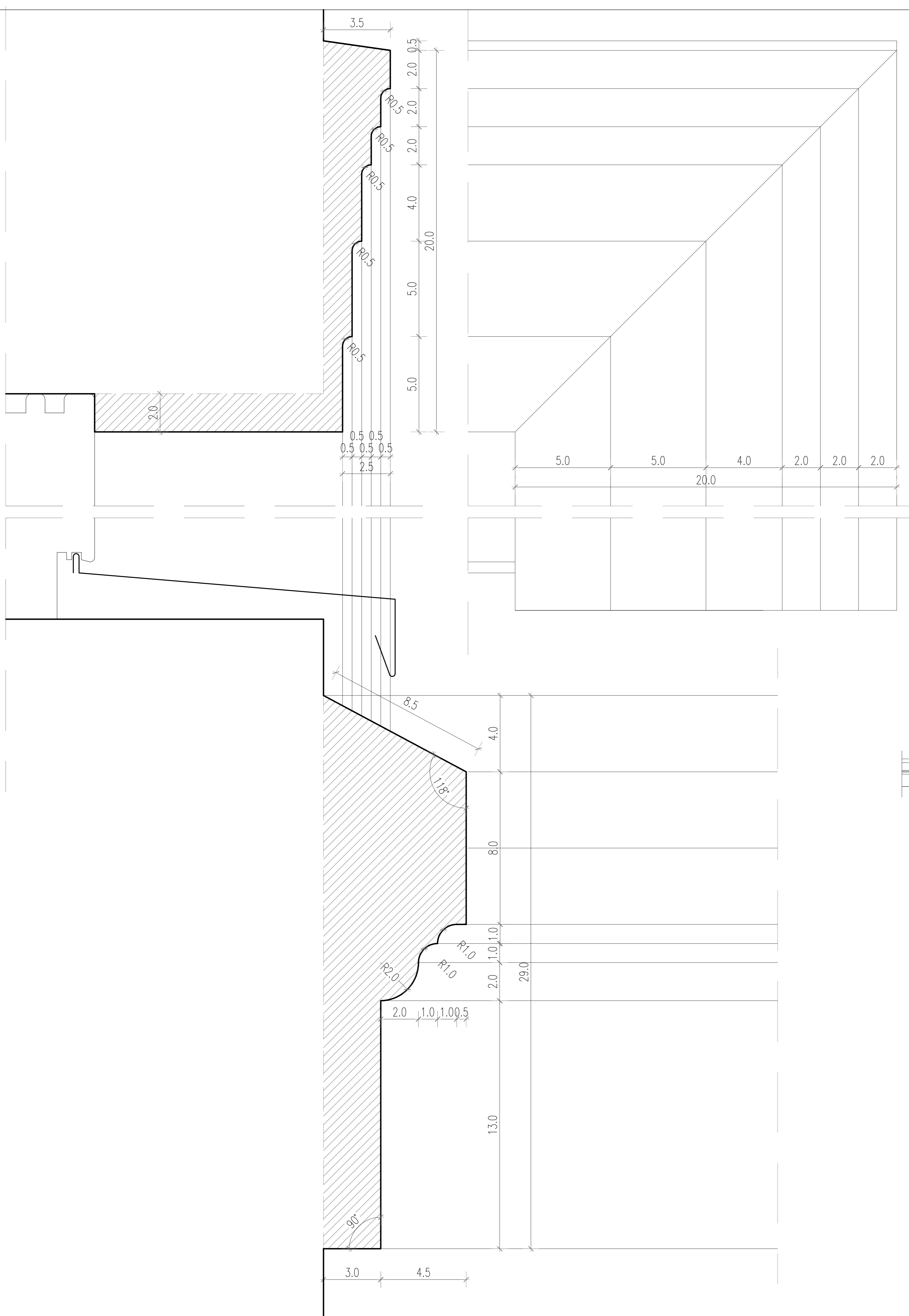
DETAL 3 Listwa wokółokienna okna 02, Parapet okna 02
