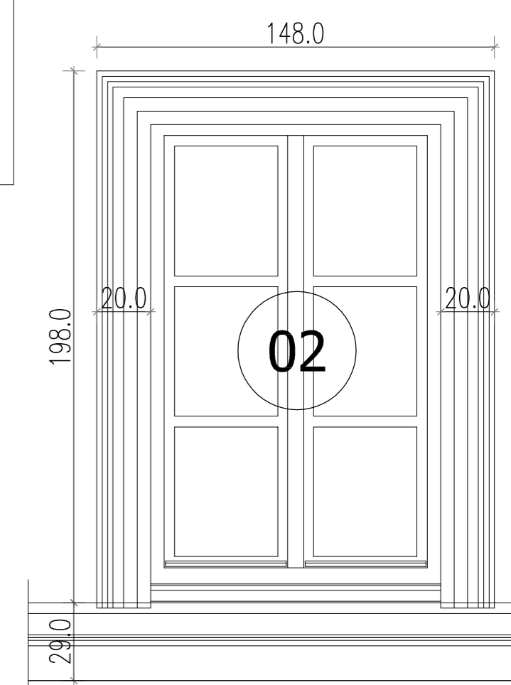
DETAL 3 Listwa wokółokienna okna 02, Parapet okna 02
