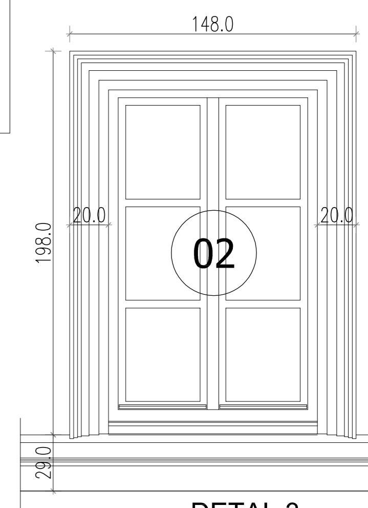
DETAL 3 Listwa wokółokienna okna 02, Parapet okna 02
