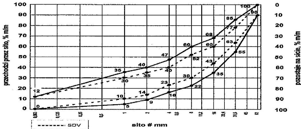
Rysunek 2. Mieszanka niezwiązana 0/63 do warstwy podbudowy pomocniczej
