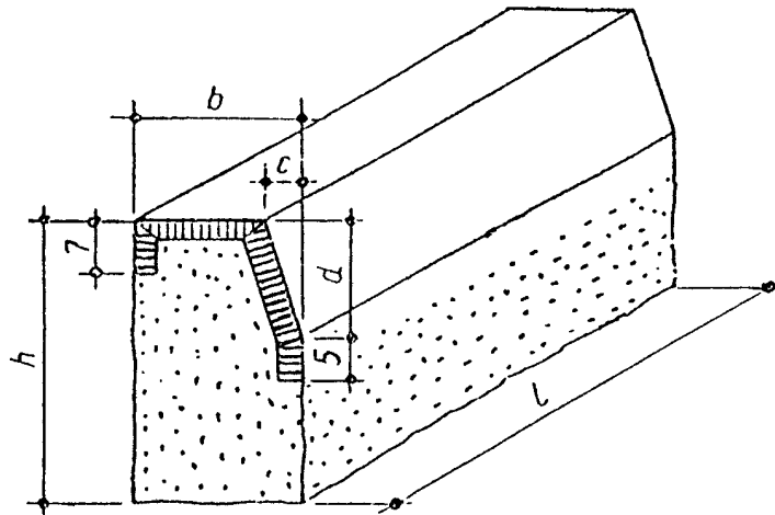
Rys. 1. Krawężnik uliczny odmiany UP, rodzaju A (nie dotyczy)
