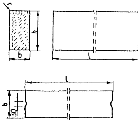
Rys. 1. Wymiarowanie krawężników
