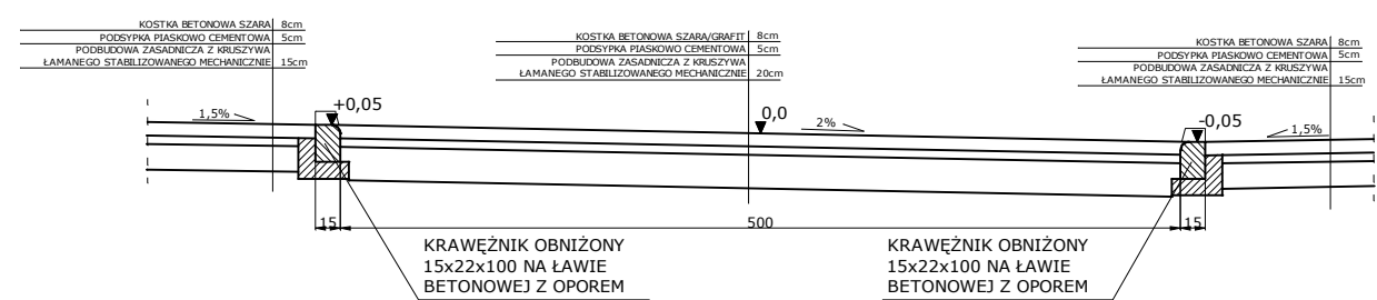
Przekrój A-A
