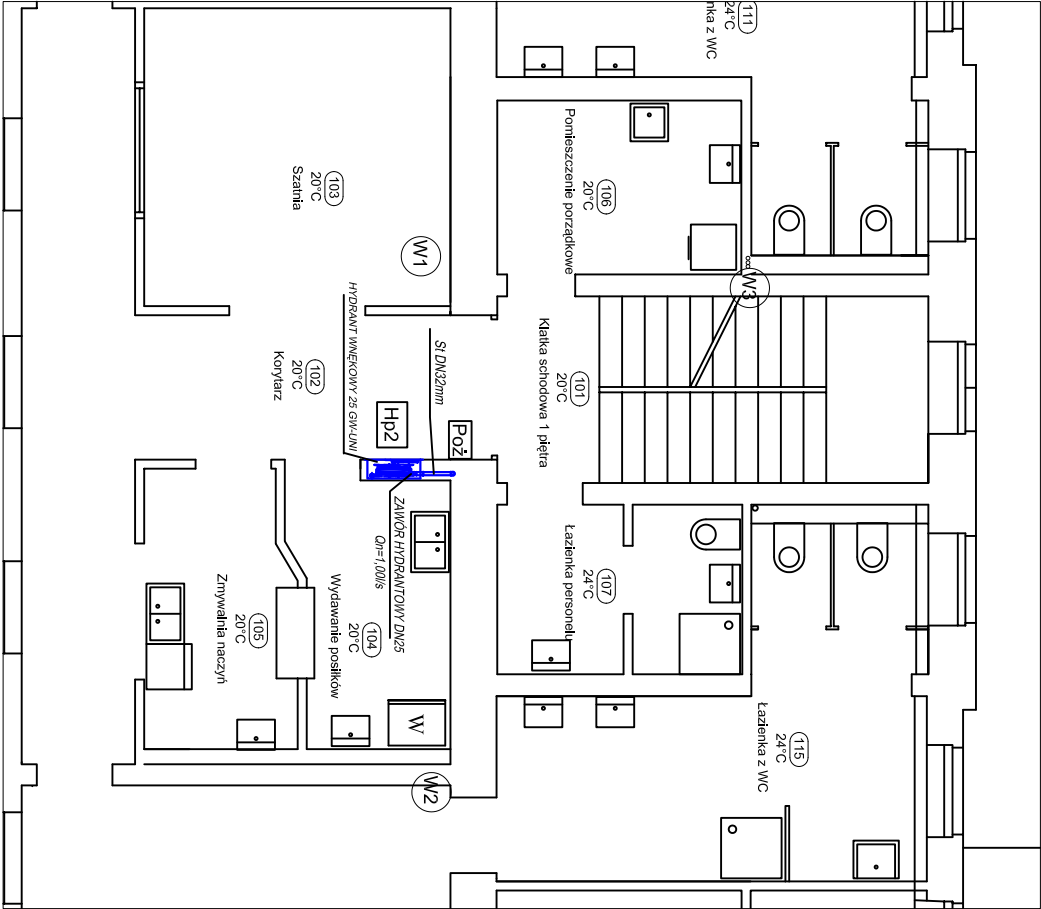
Rzut 1 Piętra 1:100
