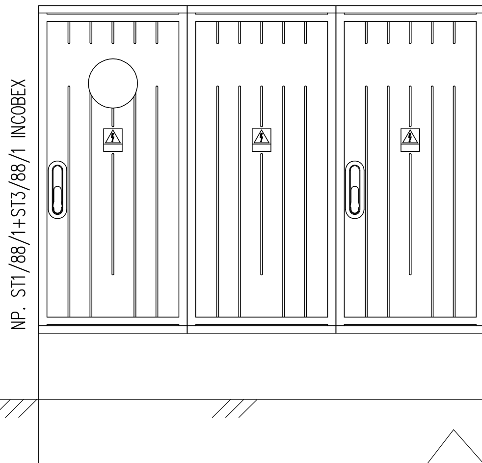
WIDOK ELEWACJI SO-863
