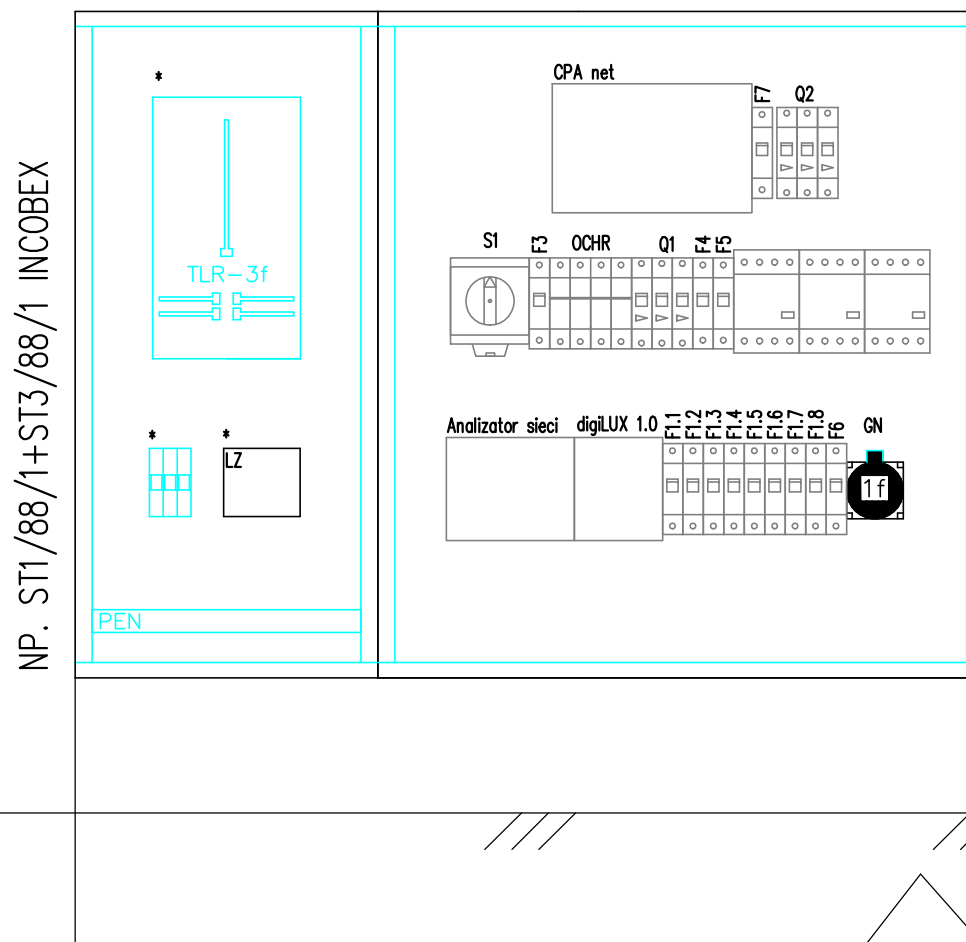
WIDOK APARATÓW SO-863
