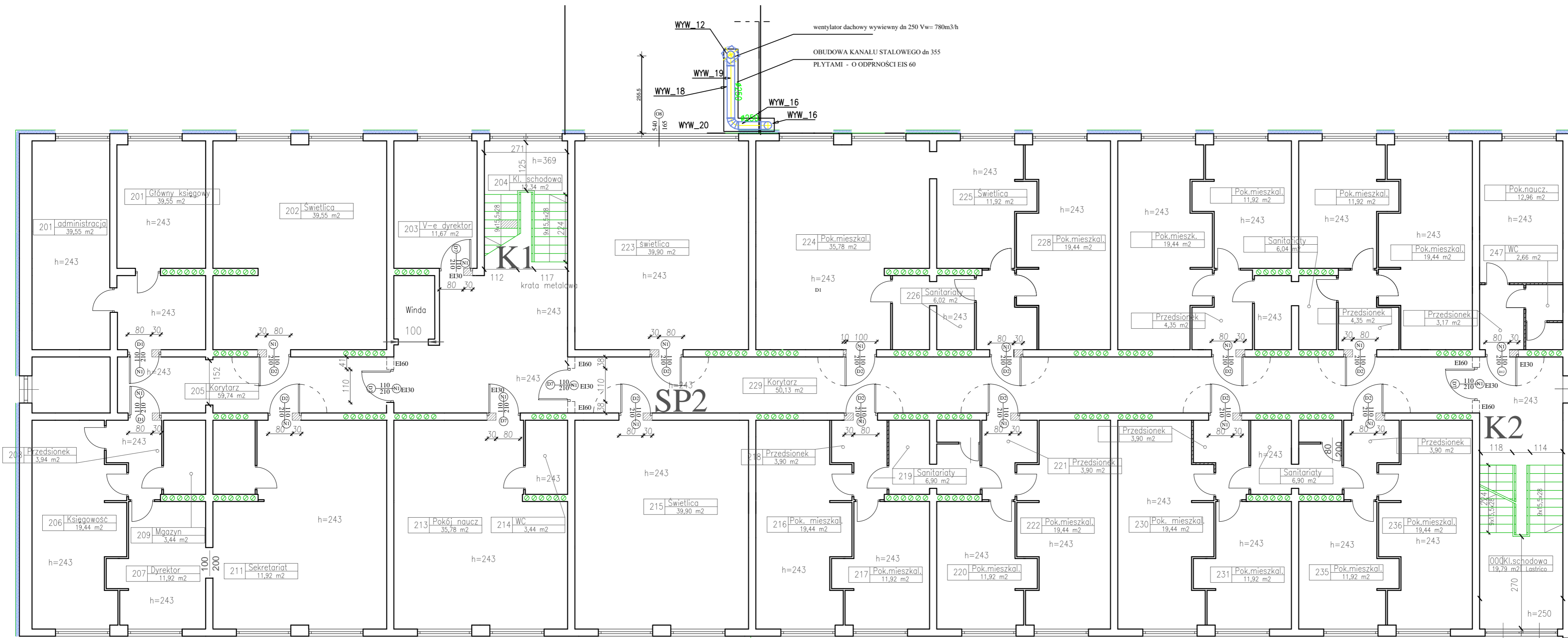
Budynek "A" - Rzut I piętra
