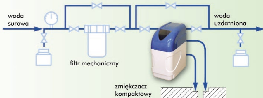
Schemat montażu stacji uzdatniania wody
