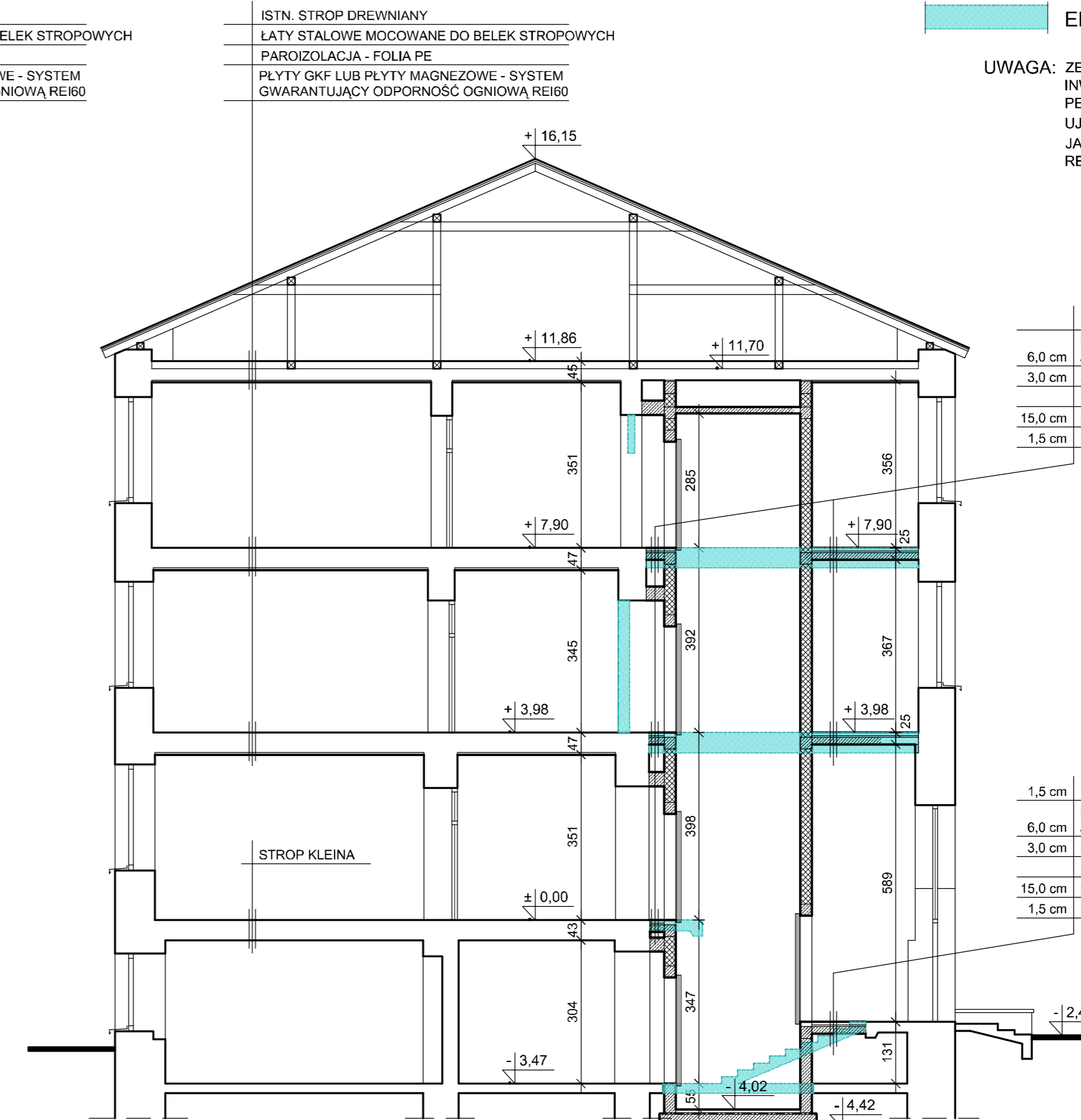
przekrój 1-1
