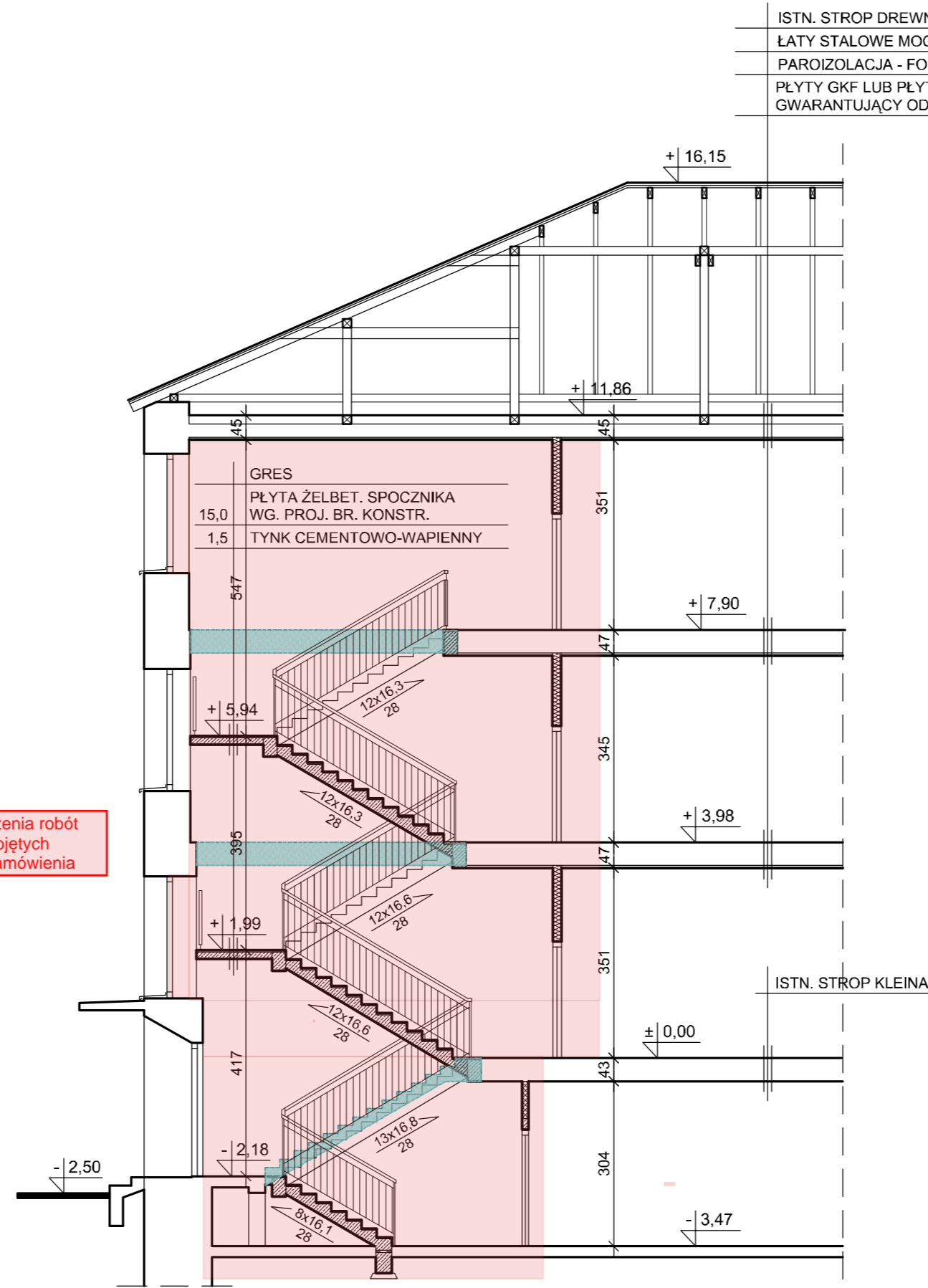
przekrój 2-2
