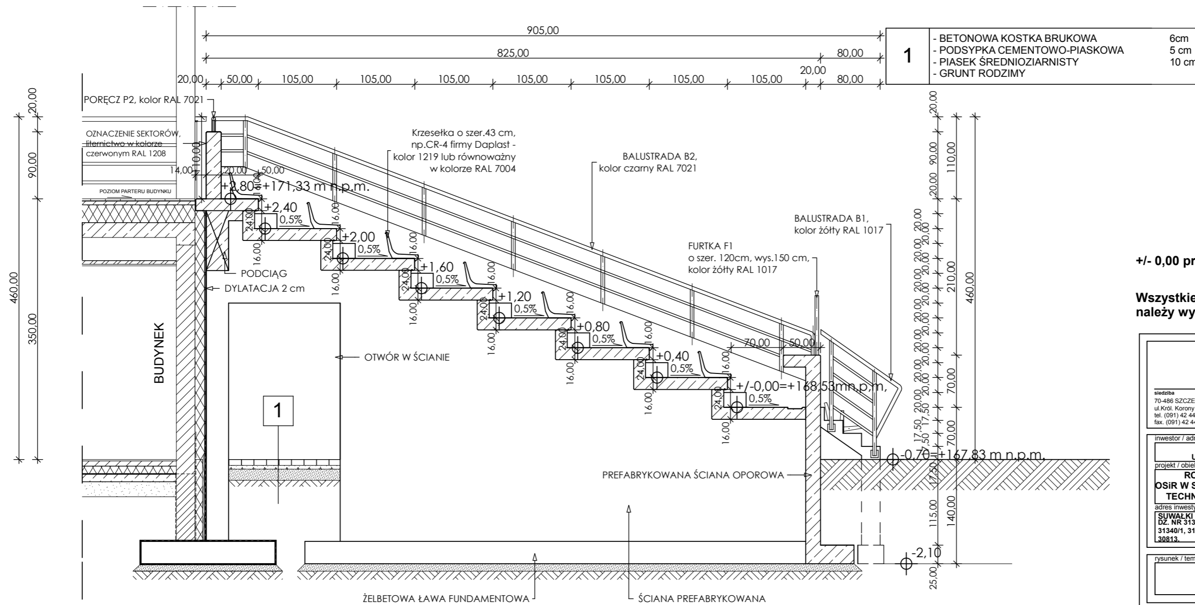
PRZEKRÓJ A - A
