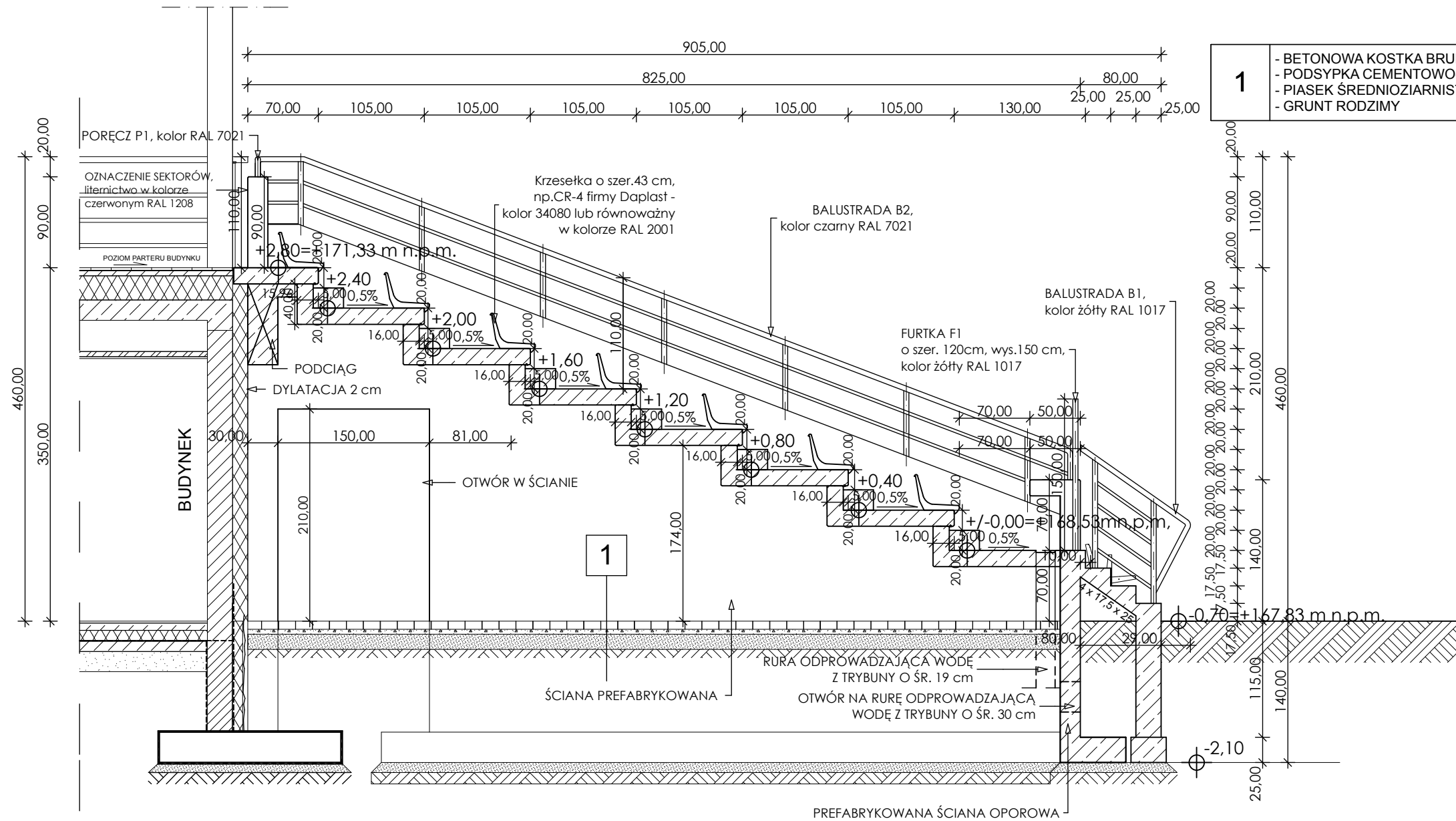
PRZEKRÓJ B - B
