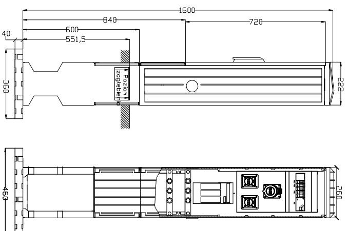
Z5 - elewacja
