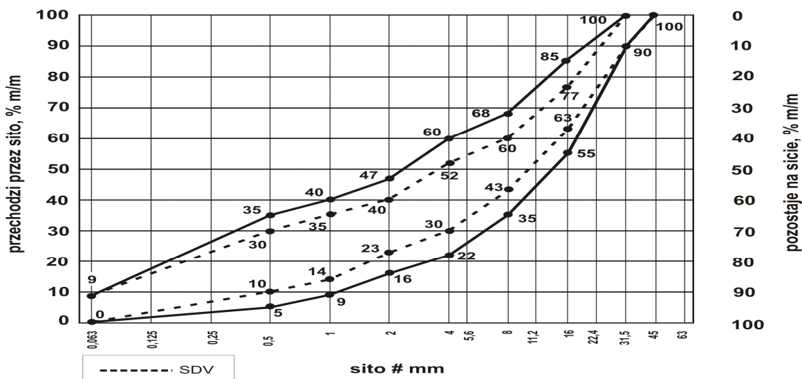
Rys. 6.4.4. Uziarnienie mieszanki niezwiązanej 0/31,5 do podbudowy zasadniczej
