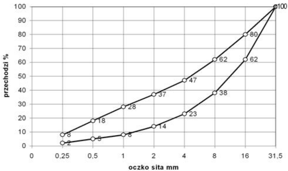
Rysunek 2. Graniczne krzywe uziarnienia kruszywa 0÷31,5 mm
