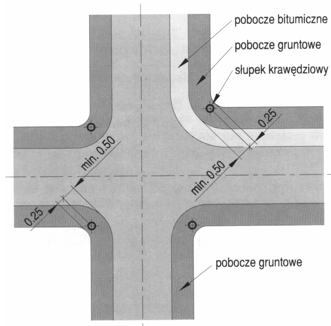
Rys. 8.2.2.2. Umieszczanie słupków krawędziowych w obrębie skrzyżowania
