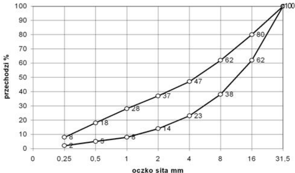
Rysunek 2. Graniczne krzywe uziarnienia kruszywa 0÷31,5 mm (dla betonu klasy C12/15 (B15) - C20/25 (B25))
