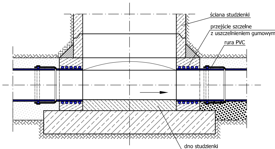
USTAWIENIE PRZEJŚĆ SZCZELNYCH KIELICHOWYCH W KOMORZE PRZEPLYWOWEJ
